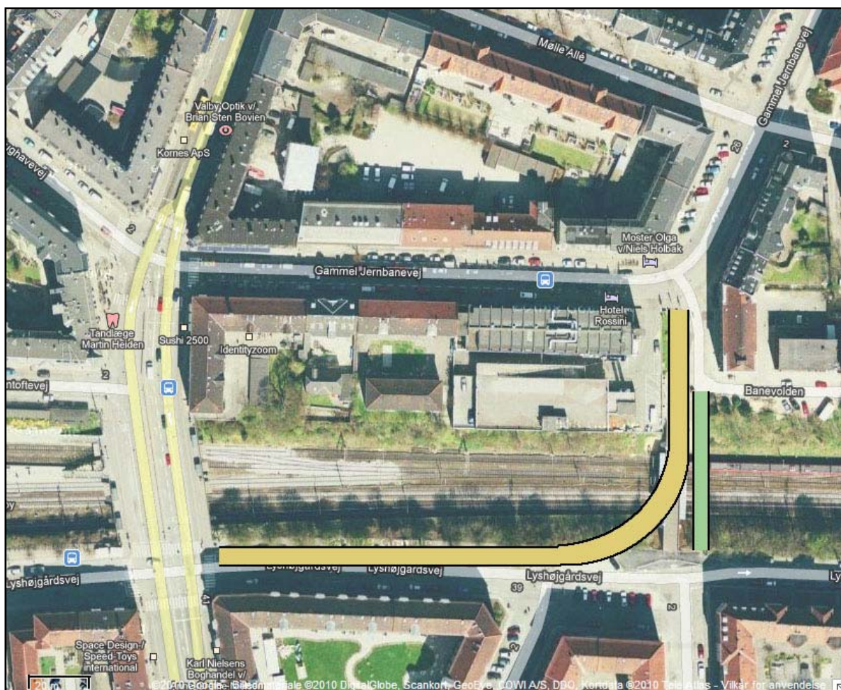
Figur 20: Skitse af det foreslåede letbanetracé med to nye broforløb over banegraven ved Banevolden
